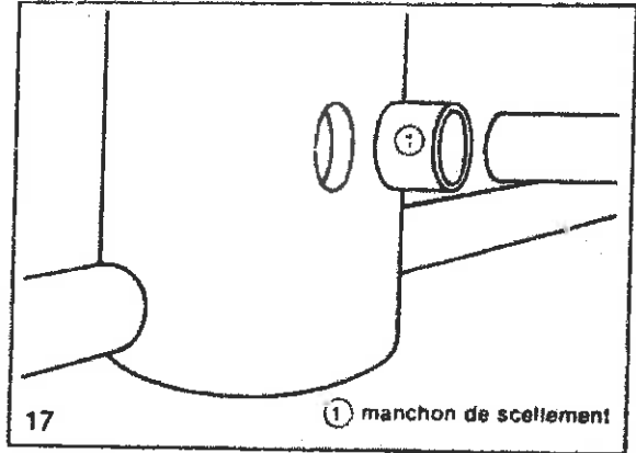
Branchement sur regard visible
