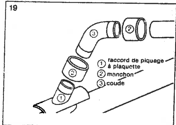
Branchement sur collecteur par plaquette
