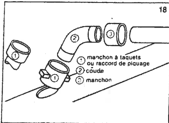
Branchement sur collecteur par piquage
